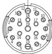
Bild 1: Polbild Buchsenstecker Ansicht auf Steckseite
