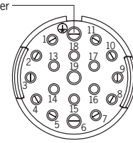
Bild 2: Polbild Buchsenstecker Ansicht auf Steckseite
