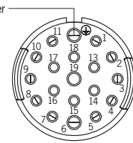
Bild 3: Polbild Stiftstecker Ansicht auf Steckseite
